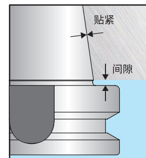
普通BT接口
