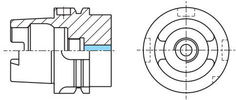
DIN 69893 - HSK-A
