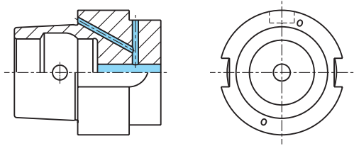
DIN 69893 - HSK-D
