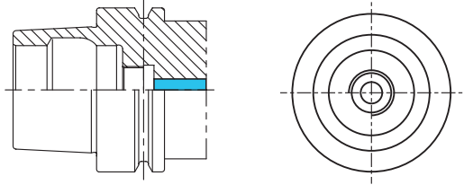
DIN 69893 - HSK-E
