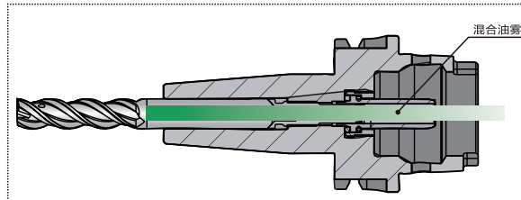
单通道自动换刀微量润滑刀柄
