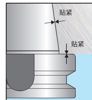
双面定位BB接口
