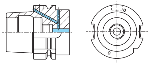
DIN 69893 - HSK-B
