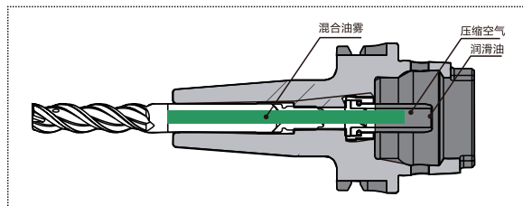
双通道自动换刀微量润滑刀柄
