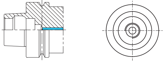
DIN 69893 - HSK-F
